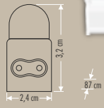
CT-2469 T5 BANT ARMATÜR BEYAZ KASA EKLENEĞİLİR ANAHTARLI
