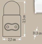
CT-2467 T5 BANT ARMATÜR BEYAZ KASA EKLENEĞİLİR ANAHTARLI
