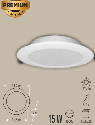
CT-5235 SIVA ÜSTÜ LED PANEL
